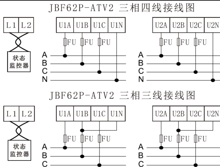
图 2 接线示意图
