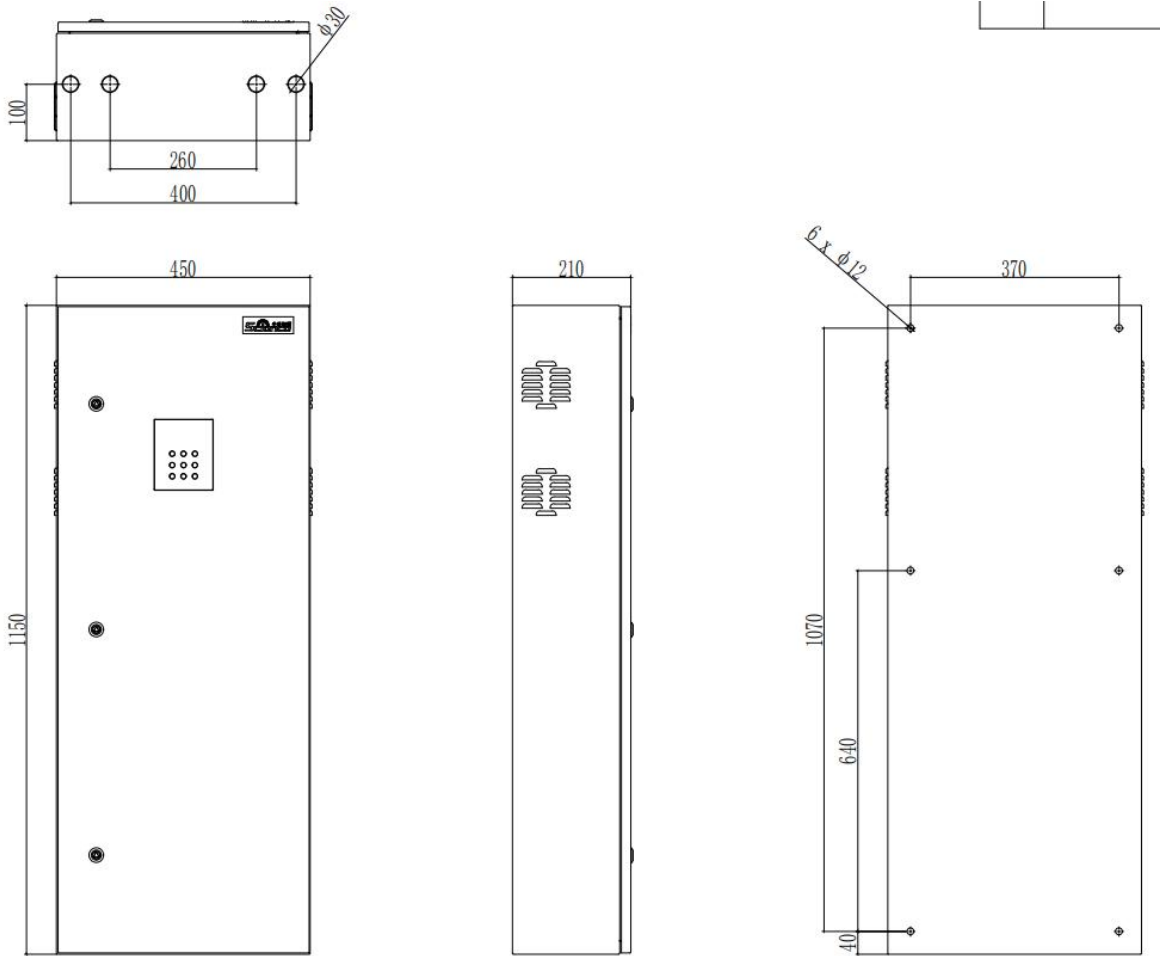
图 2.1 外形尺寸图
