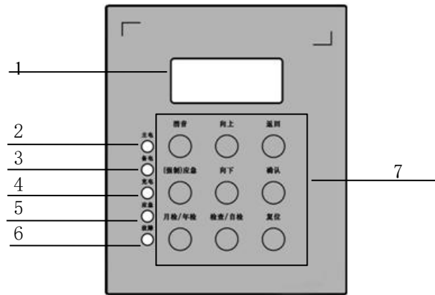
图 4.1 操作面板
