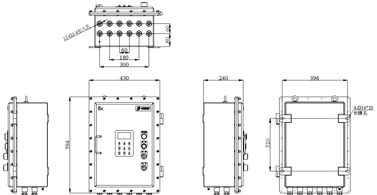
图 2.1 外形尺寸图
