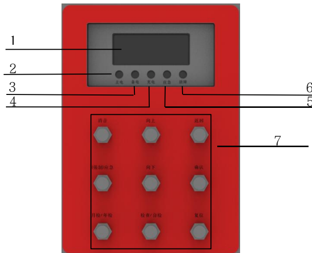
图 4.1 操作面板
